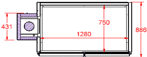
A-A ( 1 : 20 )
